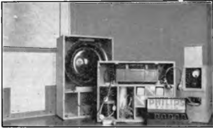
De installatie, zoals deze door de Karakorum-Expeditie gebruikt wordt.
