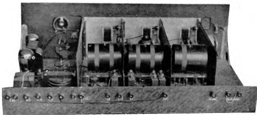
De 5 lamps aetherjager.
